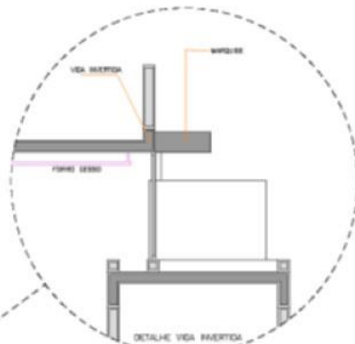
DETALHE VIGA INVERTIDA
